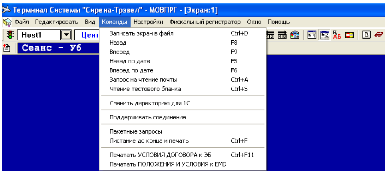
Рис. 6. Опция «Команды»
