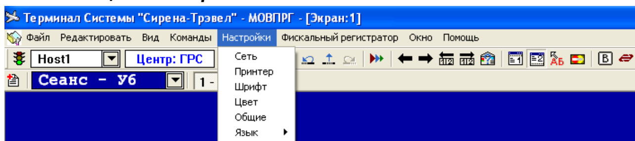
Рис. 7. Опция «Настройки»
