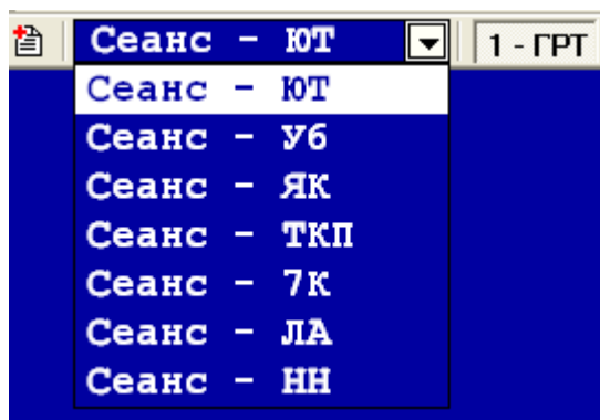
Рис. 46. Список сеансов.
