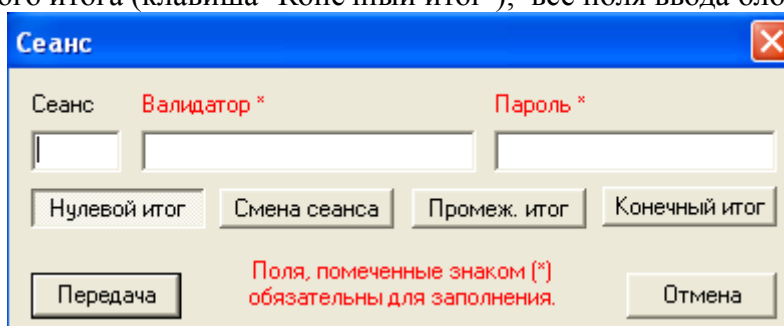
Рис. 16. Диалог «Сеанс»
