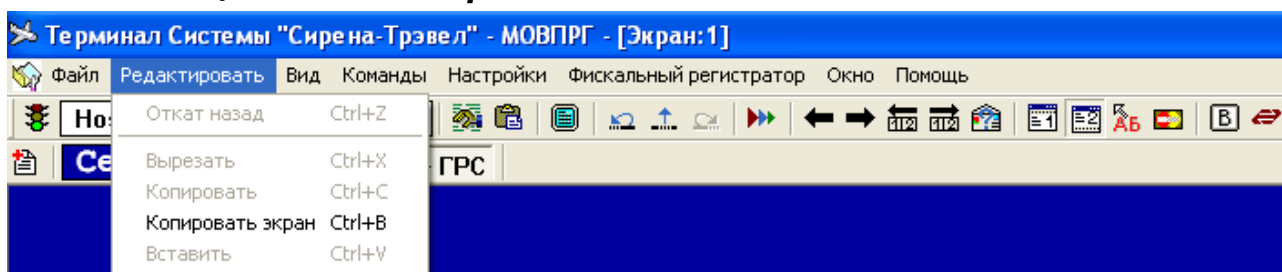
Рис. 4. Опция «Редактировать»
