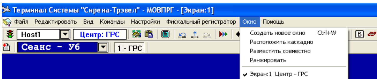
Рис. 9. Опция «Окно»
