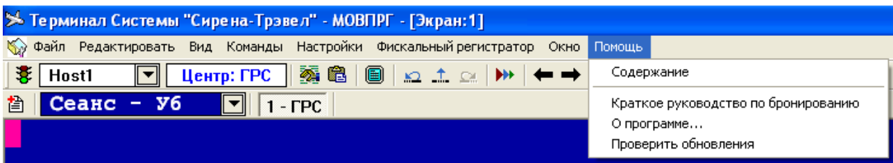
Рис. 11. Опция «Помощь»
