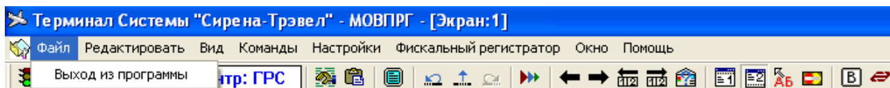
Рис. 3. Опция «Файл»
