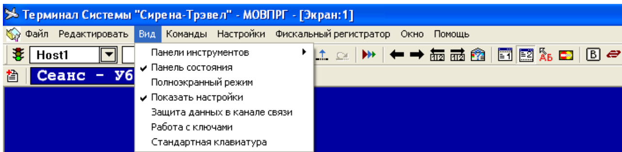
Рис. 5. Опция «Вид»
